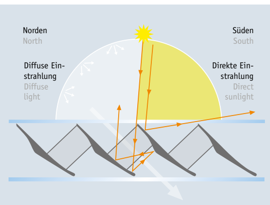
Funktionsprinzip OKASOLAR 3D (nördliche Hemisphäre) Principles of Function OKASOLAR 3D (northern hemisphere)
